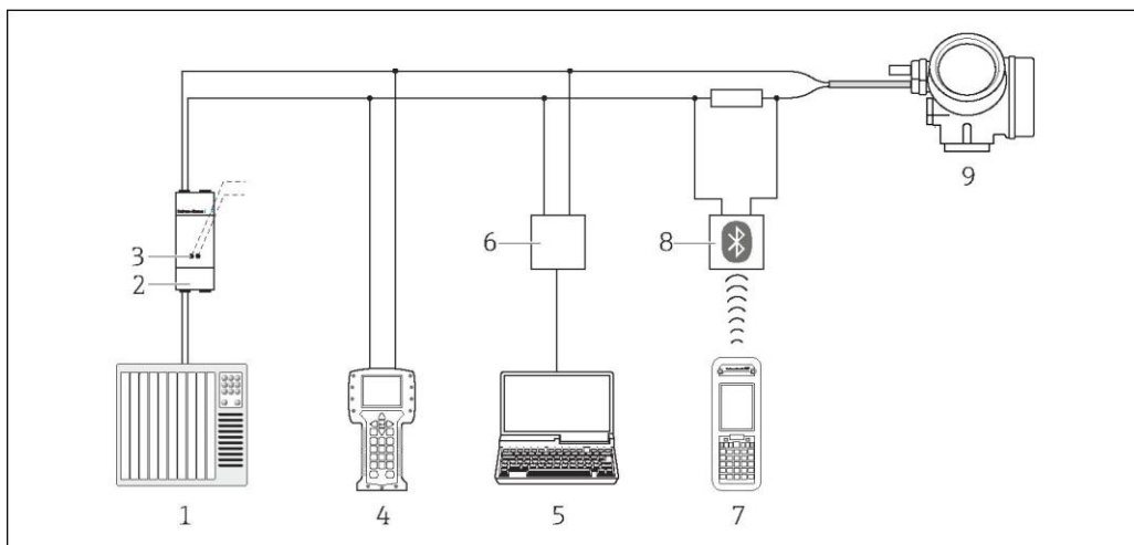
33 Варианты дистанционного управления по протоколу HART
