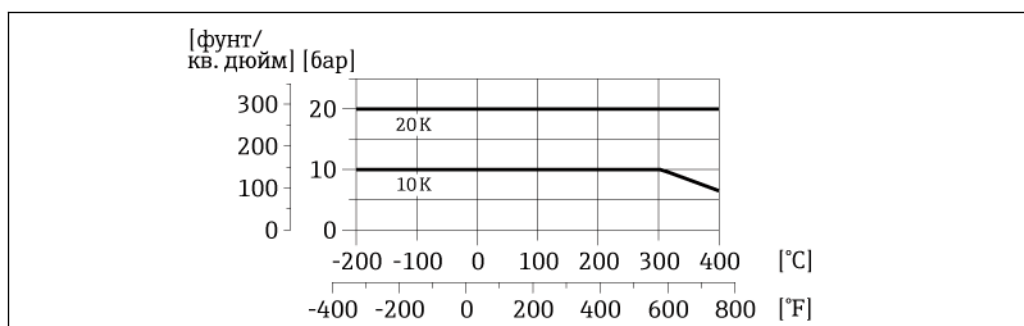
18 Материал присоединения к процессу: нержавеющая литая сталь, несколько сертификатов, 1.4404 (F316, F316L)
