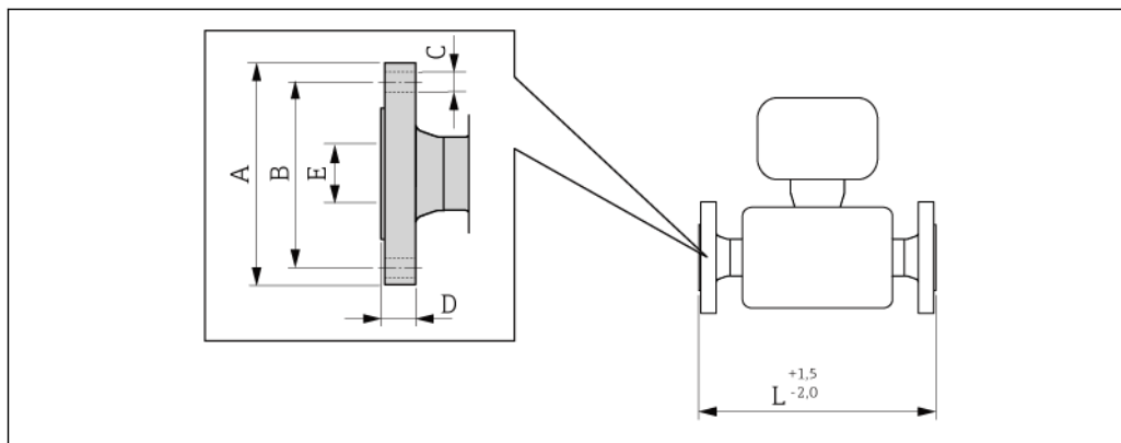
24 Единица измерения мм
