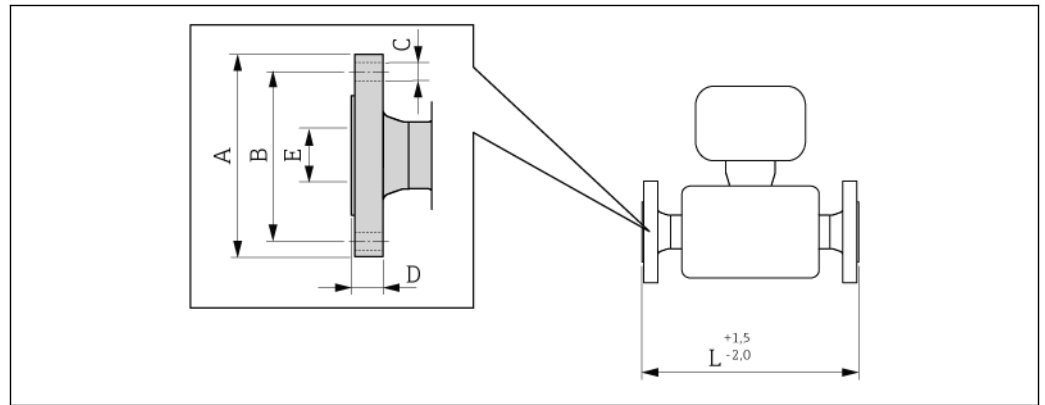
28 Единица измерения мм
