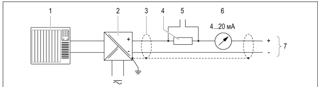
5 Пример подключения для токового выхода 4...20 мА HART (пассивный)
