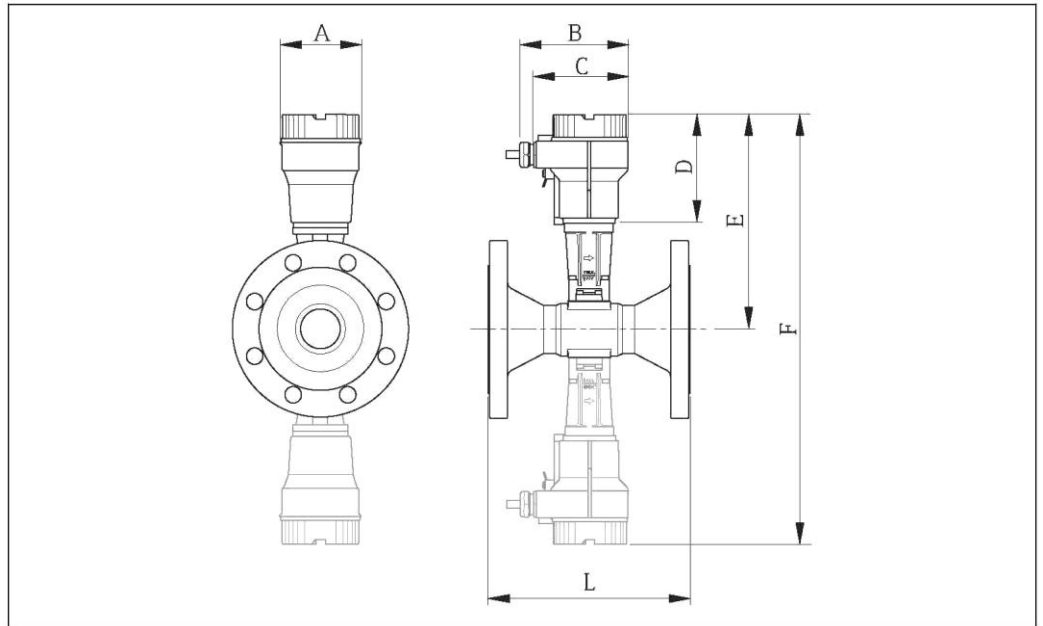
☐ 22 Серая ломаная линия: вариант исполнения Dualsens
