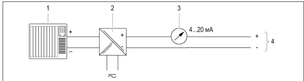
6 Пример подключения для пассивного токового выхода 4-20 мА
