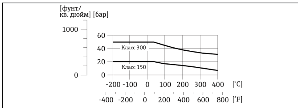
17 Материал присоединения к процессу: нержавеющая литая сталь, несколько сертификатов, 1.4404 (F316, F316L)
