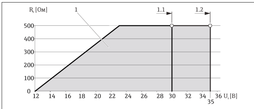
2 Нагрузка для компактного исполнения без местного управления
