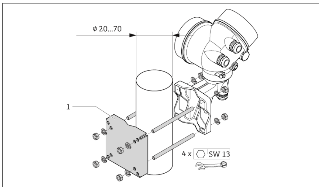
14 Единица измерения мм
