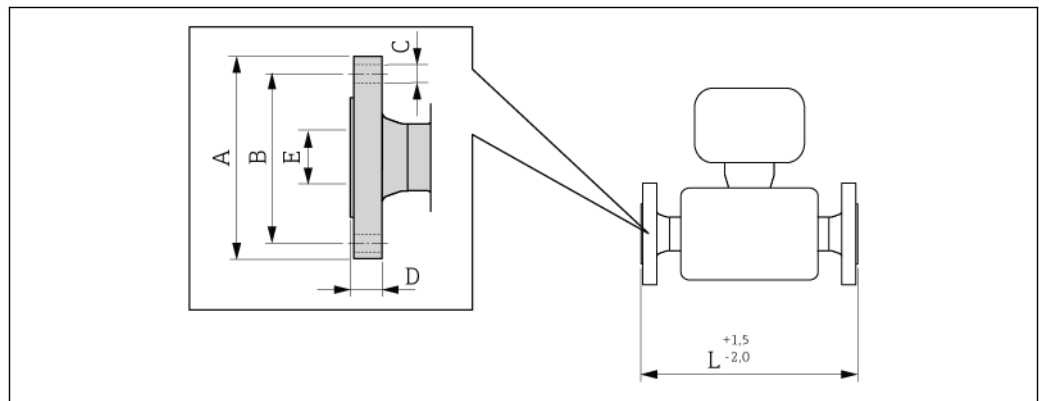
23 Единица измерения мм
