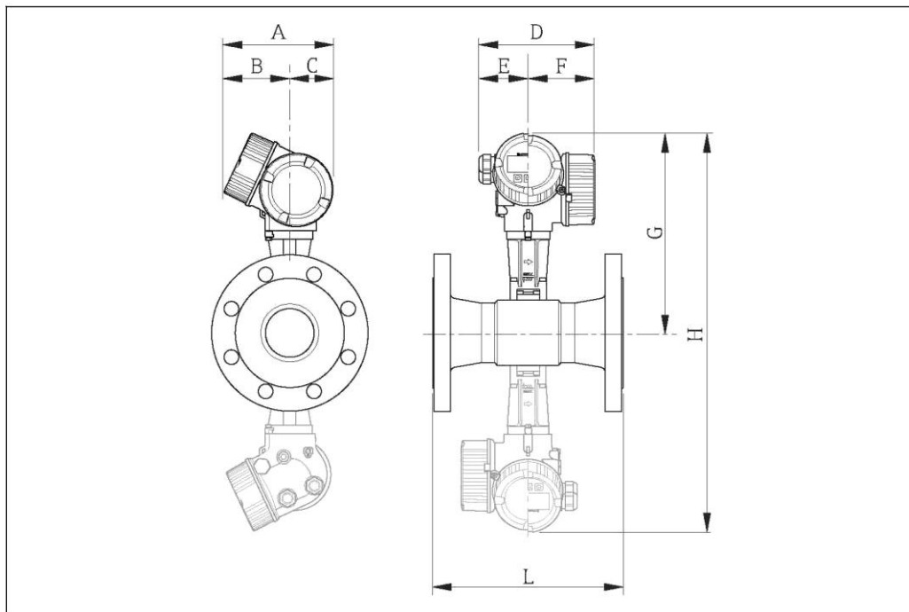
19 Серая ломаная линия: вариант исполнения Dualsens
