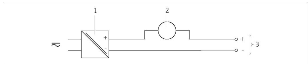
10 Пример подключения для токового входа 4...20 мА
