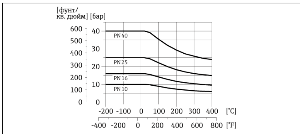
16 Материал присоединения к процессу: нержавеющая литая сталь, несколько сертификатов, 1.4404 (F316, F316L)
